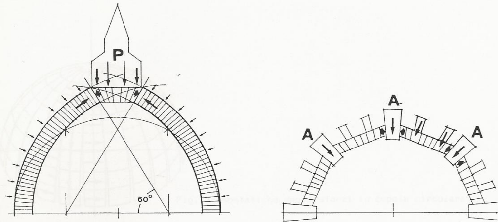
Fig.13 Trasformazione del peso dei materiali in linee di forza.
