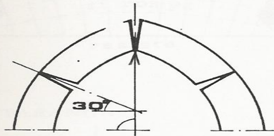
Fig.12 Apertura di lesioni in arco a sesto acuto.
