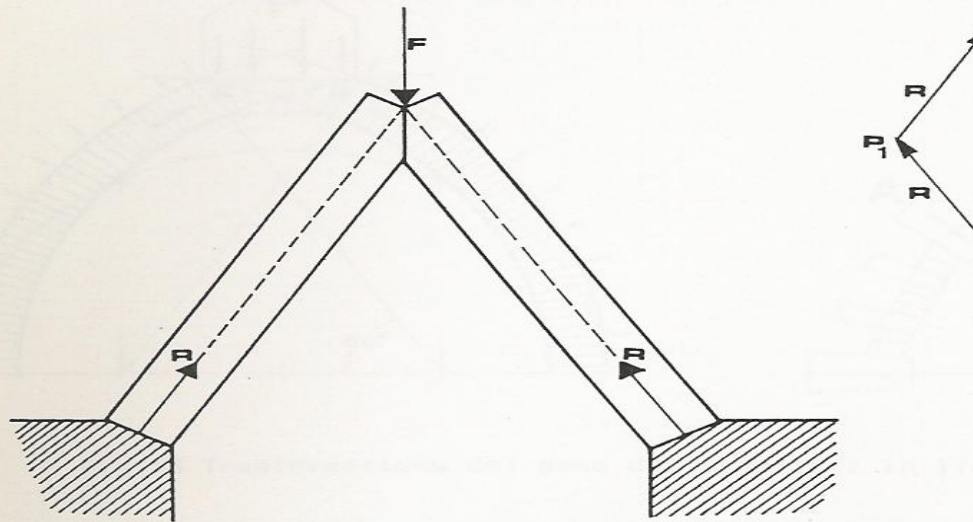
Fig.11 Portale primitivo costituito da due lastre.
